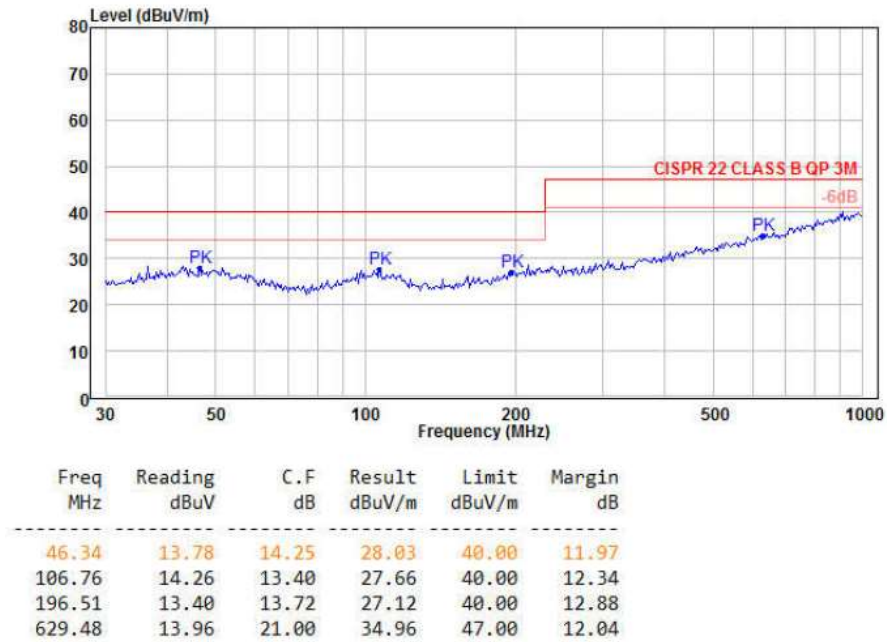
图 4-6 RE 测试垂直方向
