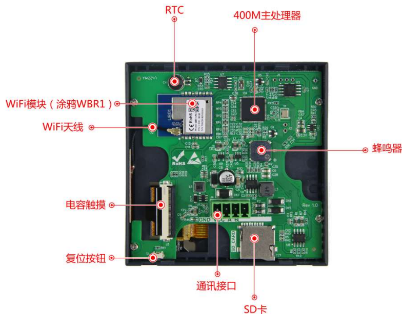
图 1-2 硬件配置图
