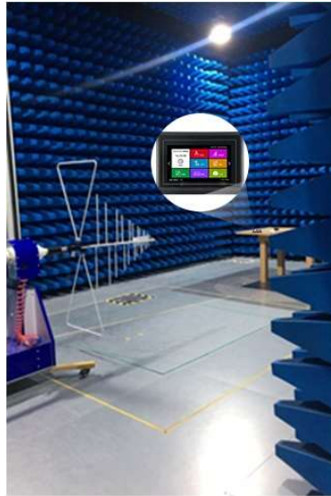
图 4-4 RE 测试图
