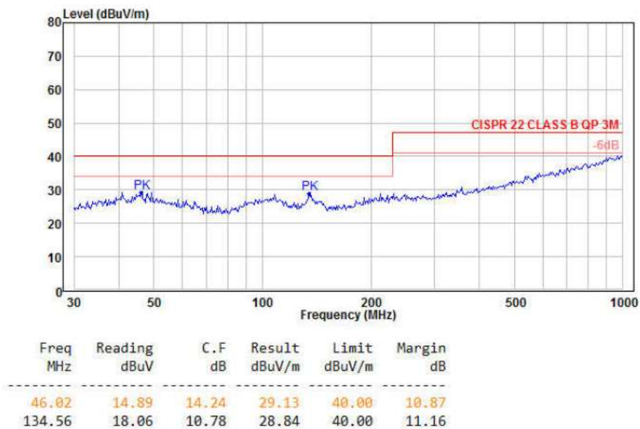
图 4-5 RE 测试水平方向
