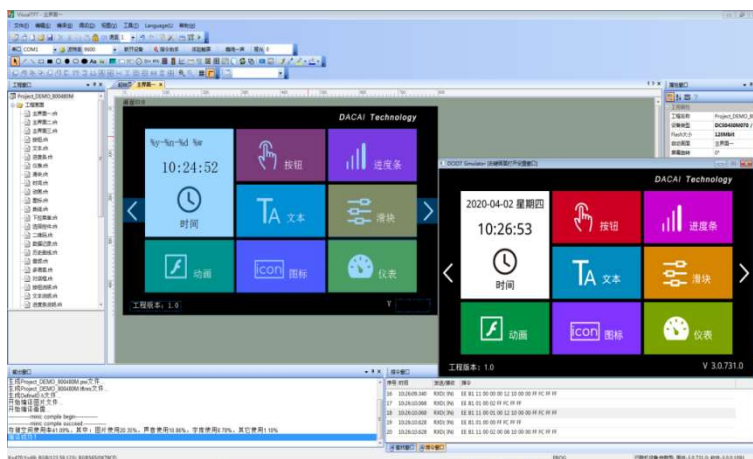
图 6-1 VisualTFT 主界面
